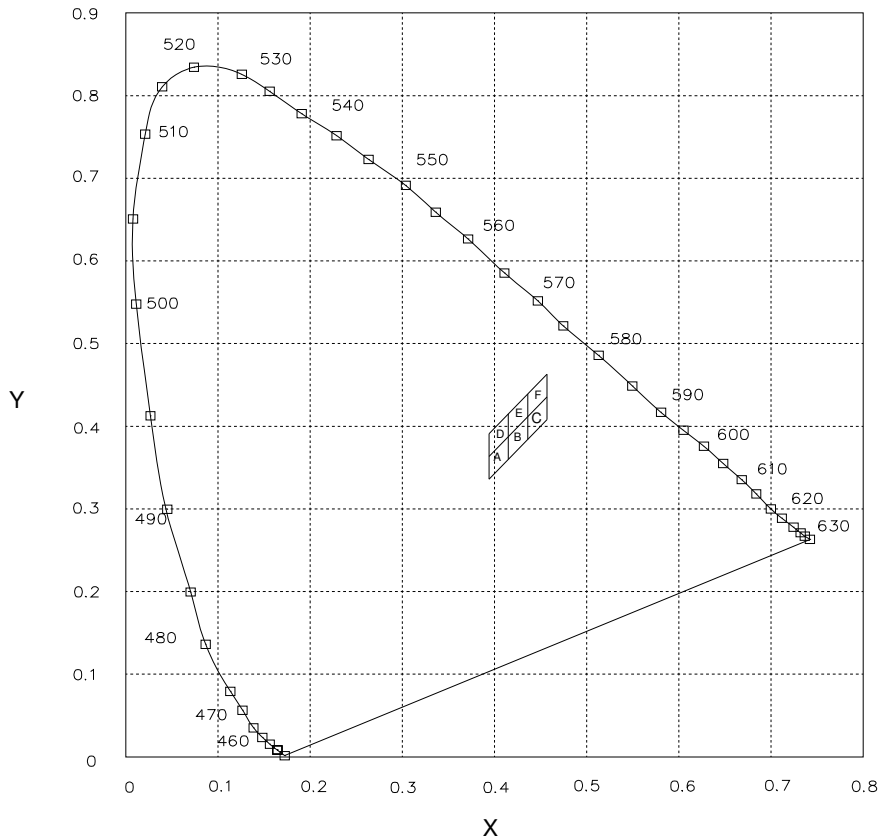
ICI Chromaticity Diagram
